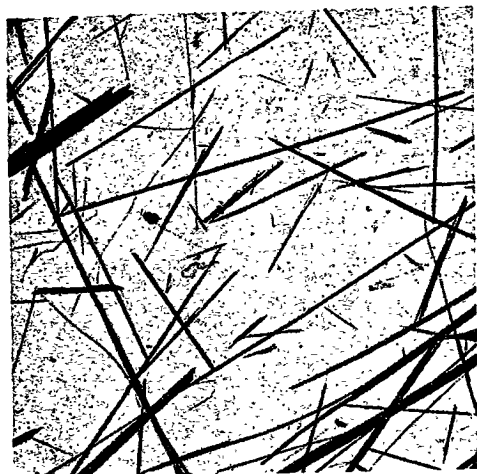
TREMOLITE 'C'
