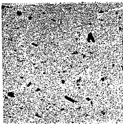
TREMOLITE 'B'
