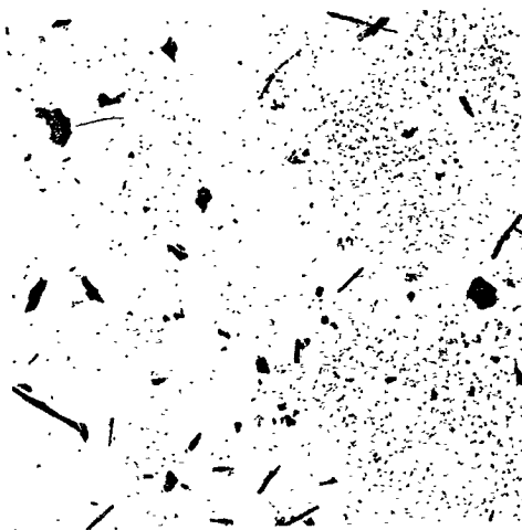
TREMOLITE 'A'
